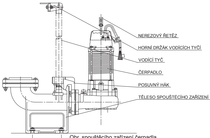
Obr. spouštěcího zařízení čerpadla
